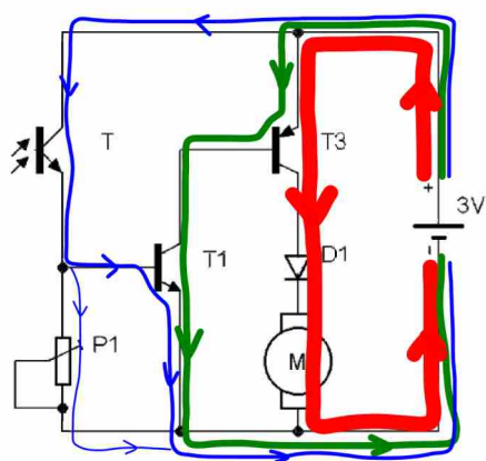
Rys. 109. Schemat ideowy Ambitnego Alberta w roli światłoluba, z zaznaczonym kolorami przepływem prądów przez poszczególne elementy
