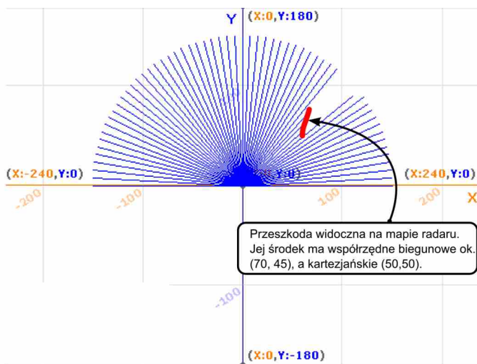
Rys. 124. Wykres odległości uzyskany przy pomocy obracającego się czujnika
