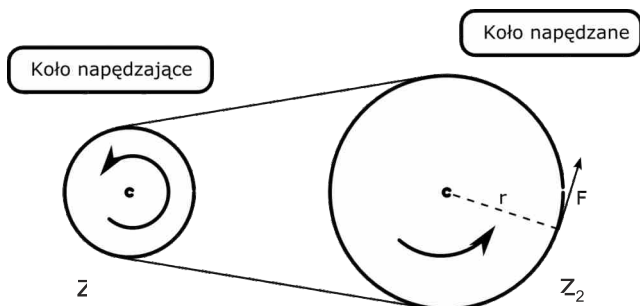
Rys. 82. Przekładnia zwiększająca moment obrotowy
