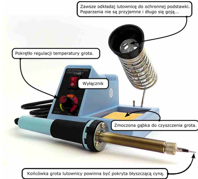
Rys. 101. Stacja lutownicza Zd99
