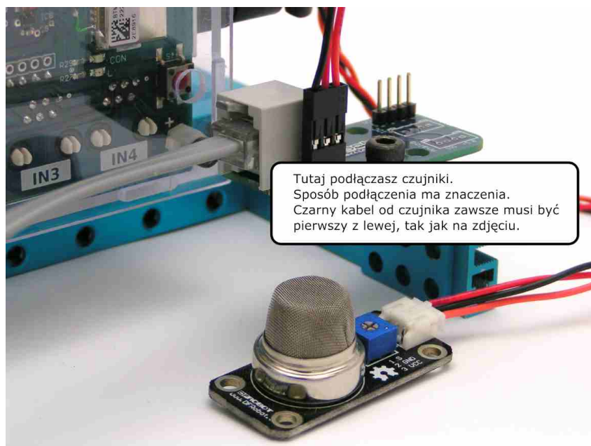
Rys. 128. Czujnik gazu podłączony za pośrednictwem interfejsu do sterownika SZM
