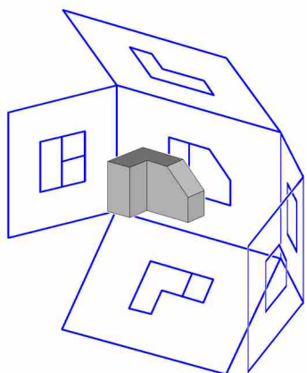
Rys. 89. Po narysowaniu wszystkich rzutów „rozwijamy” rzutnie do postaci płaskiego rysunku. Źródło: Wikimedia Commons
