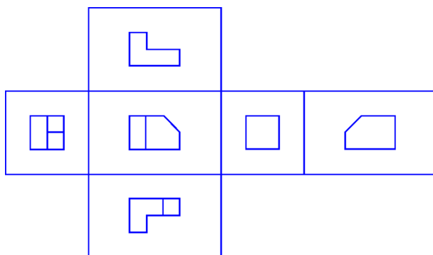
Rys. 90. Powstały w ten sposób rysunek przedstawia obiekt widziany z każdej strony. Źródło: Wikimedia Commons
