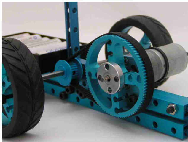
Rys. 83. Przekładnia wykonana z elementów zestawu SZM
