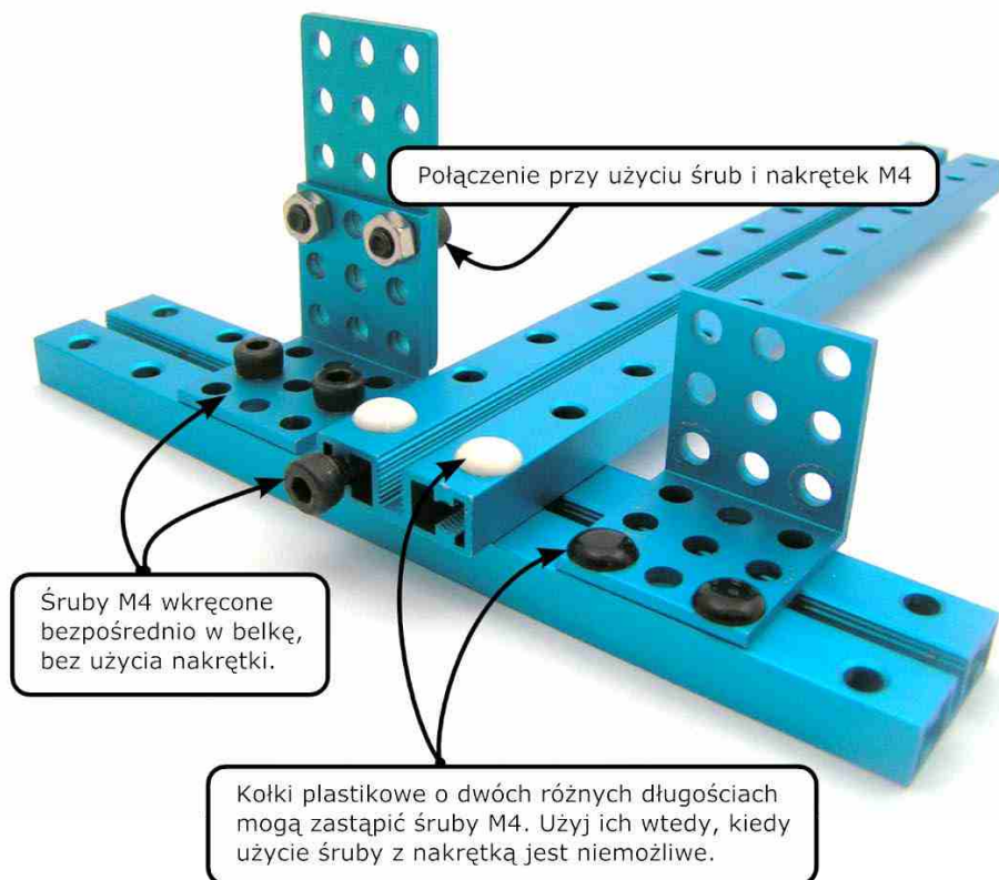
Rys. 66. Sposoby łączenia elementów zestawu SZM
