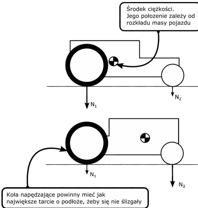
Rys. 132. Położenie środka ciężkości wpływa na nacisk wywierany przez poszczególne koła, a w konsekwencji na ich tarcie o podłoże
