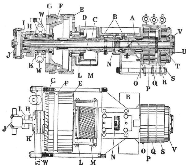
Rys. 85. Rysunek skrzyni biegów z książki „The book of motor car” wydanej w 1912 roku. Źródło: Wikimedia Commons
