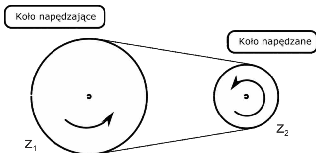
Rys. 81. Przekładnia pasowa lub łańcuchowa zwiększająca prędkość obrotową
