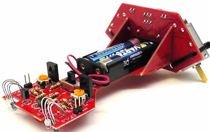
Rys. 105. Ambitny Albert - robot podążający za światłem. Widok zmontowanego robota
