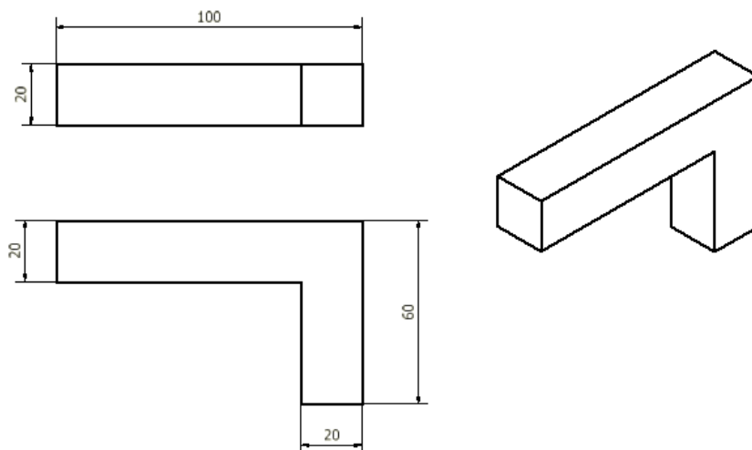
Rys. 96. Przedmiot zwymiarowany zgodnie z zasadami. Zwróć uwagę że na rysunku przedstawione są tylko dwa rzuty, wystarczające do dokładnego odwzorowania przedmiotu
