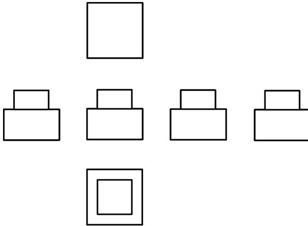
Rys. 91. Rzuty obiektu, który ma 4 takie same ściany. W tym przypadku możemy rzutować tylko front obiektu
