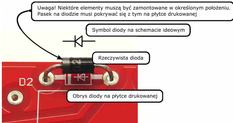
Rys. 102. Dioda D2 przygotowana do przyłutowania do płytki drukowanej
