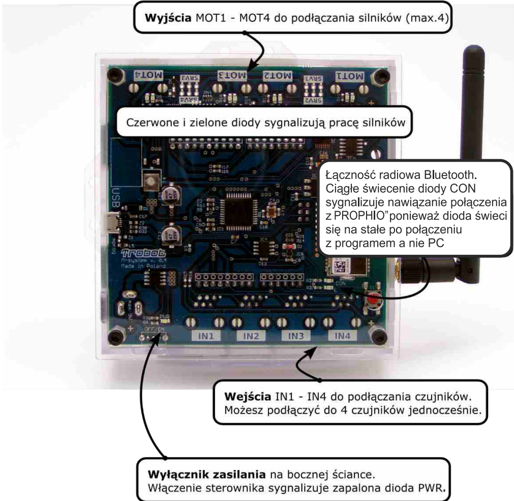
Rys. 67. Sterownik programowalny zestawu SZM widziany z góry
