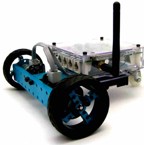
Rys. 70. Robot złożony z szkolnego zestawu mechatronicznego (SZM)
