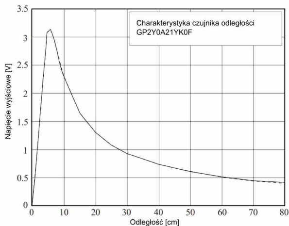
Rys. 121. Charakterystyka czujnika odległości Sharp GP2Y0A21YK0F.
