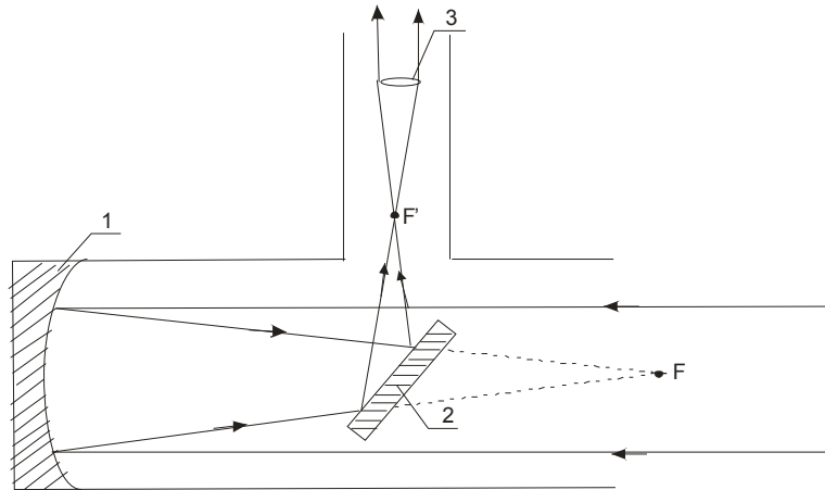
Rys.4. Schemat teleskopu Newtona (1 –główne zwierciadło paraboliczne, płaskie zwierciadło, okular)
