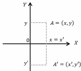
Rysunek 1-3. Symetria względem osi OX
