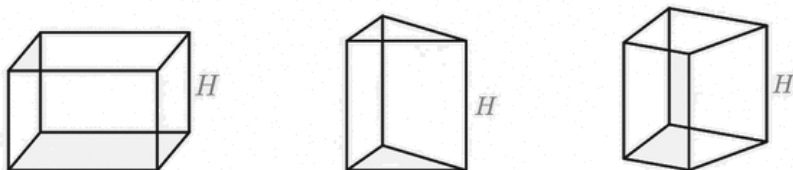
Rysunek 4-10. Gnaniostłupy proste
