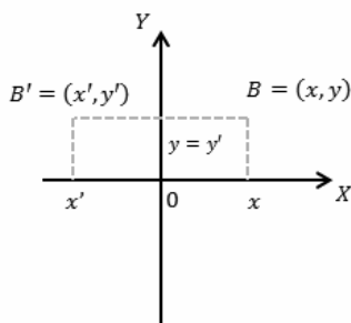
Rysunek 1-4. Symetria względem osi OY
