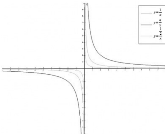
Rysunek 3-1. Wykres funkcji hiperbolicznej, a > 0
