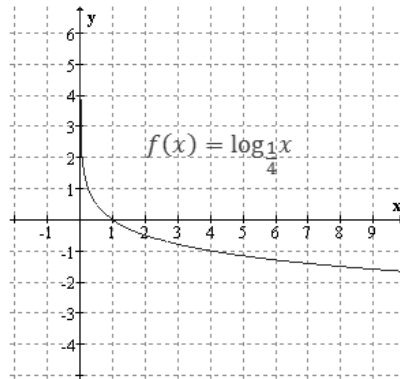
Rysunek 3-12. Wykresy funkcji logarytmicznych, 0 < a < 1
