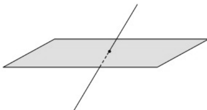
Rysunek 4-4. Prosta przecinająca płaszczyznę
