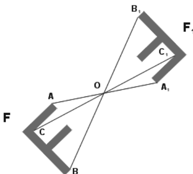
Rysunek 1-5. Przykład figury środkowosymetrycznej4
