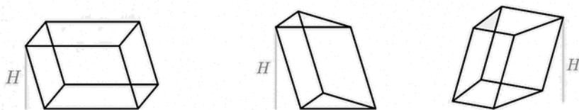
Rysunek 4-11. Gnaniostłupy pochyłe
