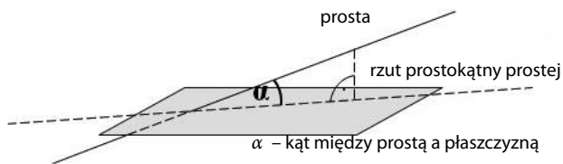
Rysunek 4-7 Kąt między płaszczyzną a prostą
