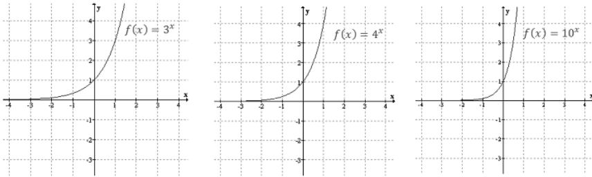
Rysunek 3-6. Wykresy funkcji wykładniczych, a > 0
