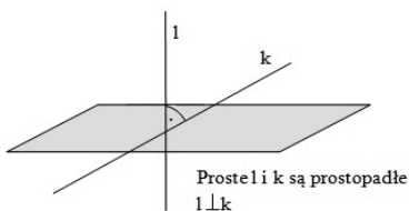
Proste prostopadłe przecinające się
