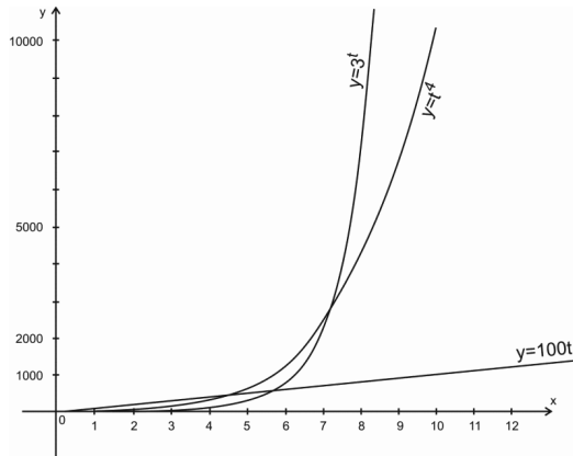
Rysunek 3-13. Wzrost wykładniczy
