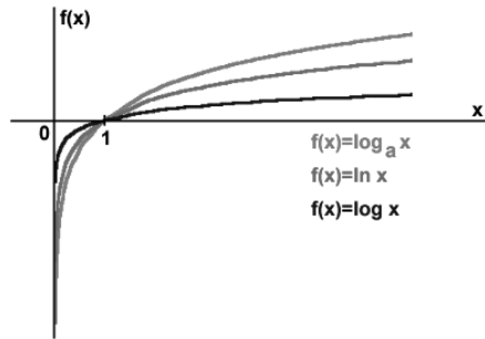
Rysunek 3-10. Wykres funkcji logarytmicznej przy podstawie e
