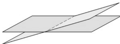
Rysunek 4-2. Płaszczyzny przecinające się
