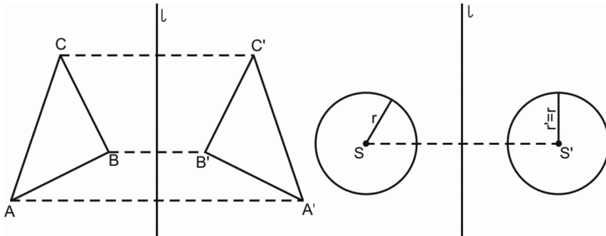
Rysunek 1-1. Przykłady figur symetrycznych
