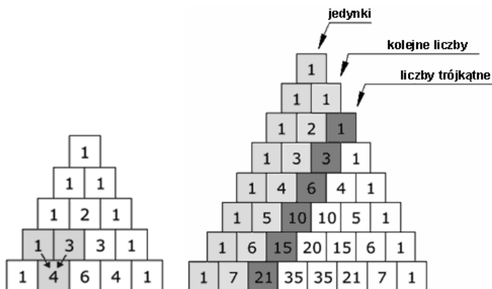
Rysunek 2-2. Zasada tworzenie trójkąta Pascala
