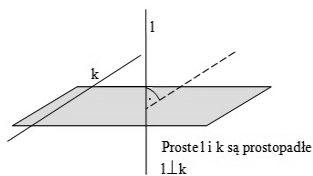
Proste prostopadłe skośne
