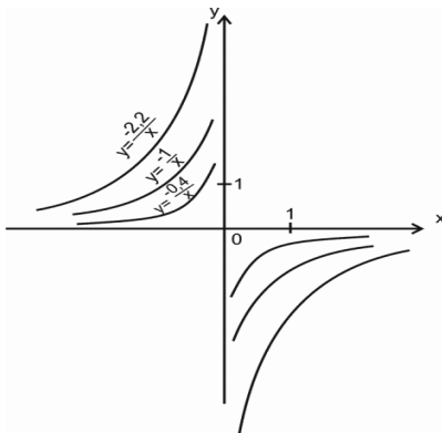
Rysunek 3-4. Wykresy funkcji f(x) = \frac{a}{x} , a < 0
