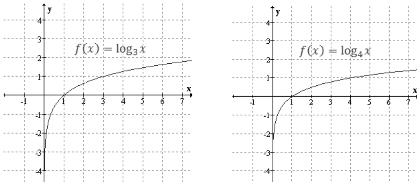
Rysunek 3-11. Wykres funkcji logarytmicznych, a > 1
