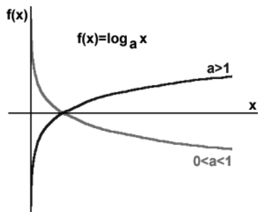
Rysunek 3-8. Wykresy funkcji logarytmicznych
