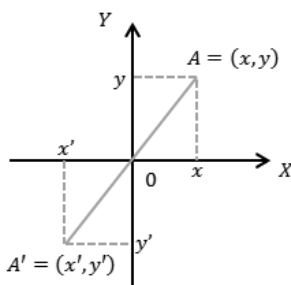
Rysunek 1-6. Symetria względem punktu (0,0)
