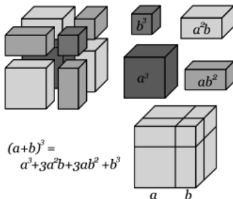
Rysunek 2-1. Graficzne uzasadnienie wzoru na sześcian sumy 24
