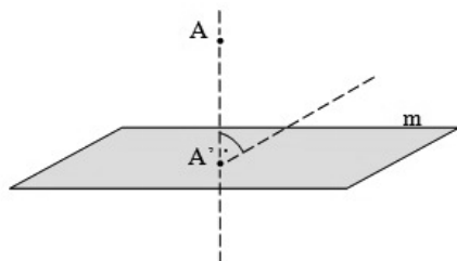
Rysunek 4-6. Rzut prostokątny na płaszczyznę
