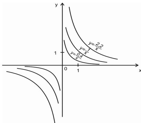
Rysunek 3-3. Wykresy funkcji f(x) = \frac{a}{x} , a > 0
