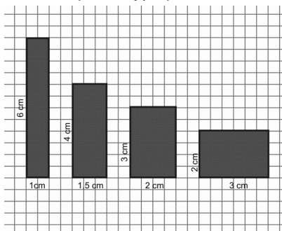
Rysunek 3-5. Prostokąty o równym polu
