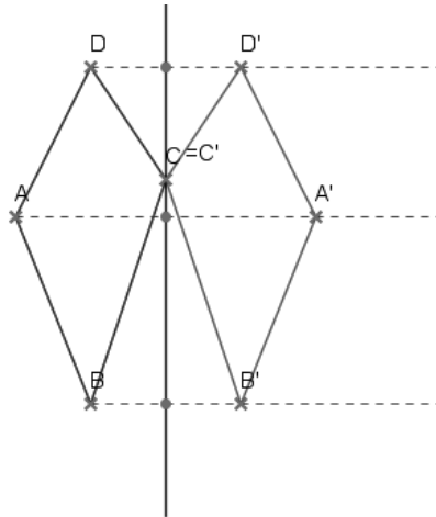
Rysunek 1-2. Figury symetryczne
