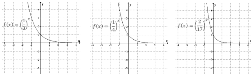
Rysunek 3-7. Wykresy funkcji wykładniczych, a < 0
