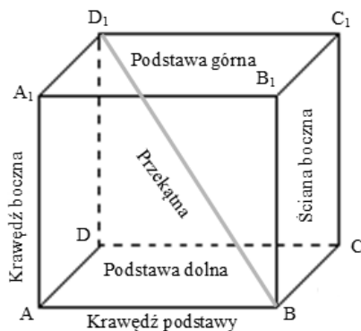
Rysunek 4-9. Gnaniostłup prawidłowy
