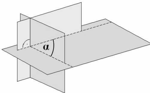
Rysunek 4-8. Kąt dwuścienny
