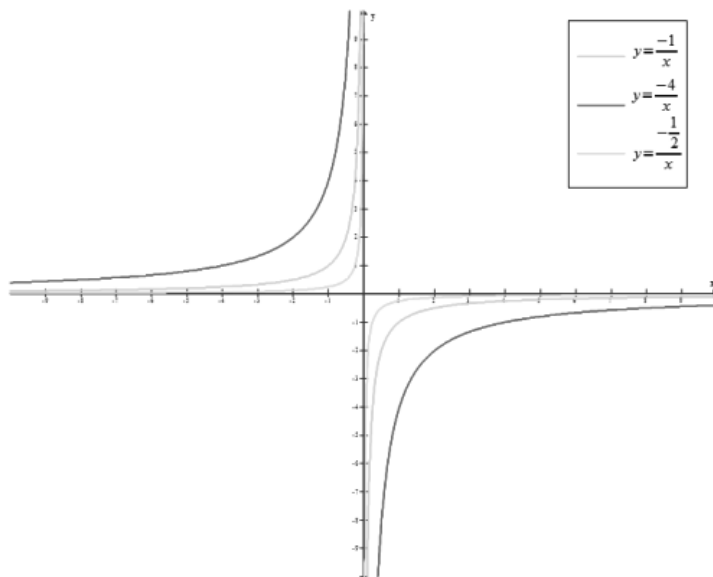
Rysunek 3-2. Wykres funkcji hiperbolicznej, a < 0
