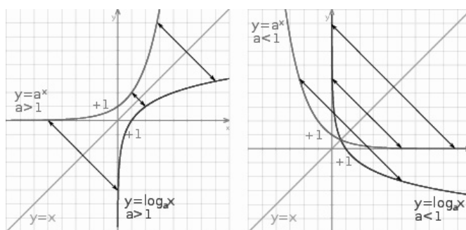
Rysunek 3-9. Funkcja wykładnicza a logarytmiczna
