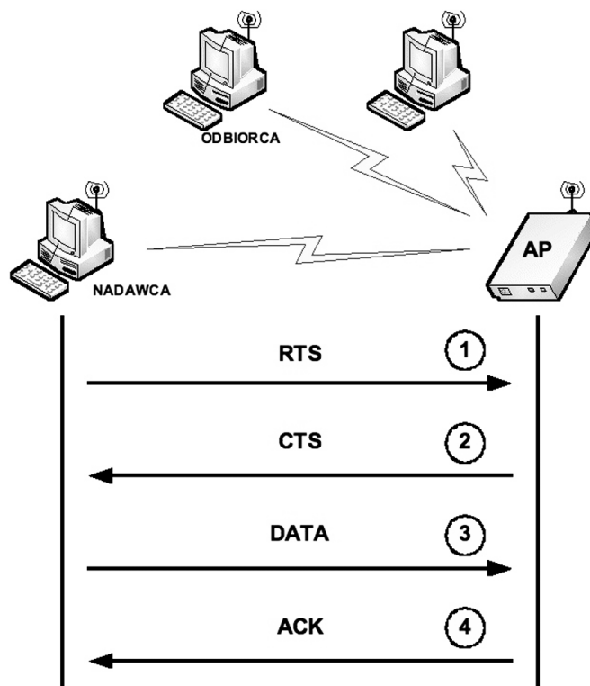
Rysunek 8. Schemat działania metody CSMA/CA
