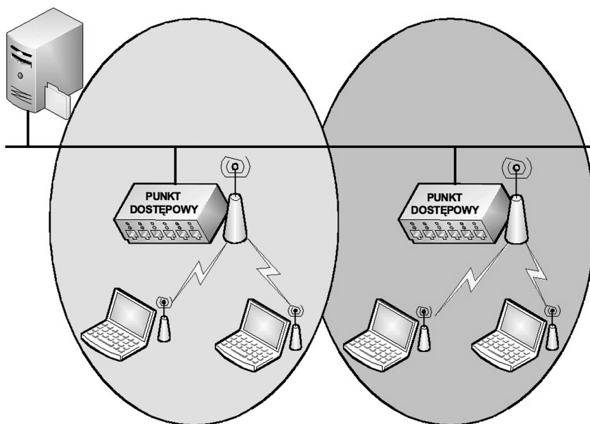
Rysunek 7. Technologia sieci infrastrukturalnej ESS
