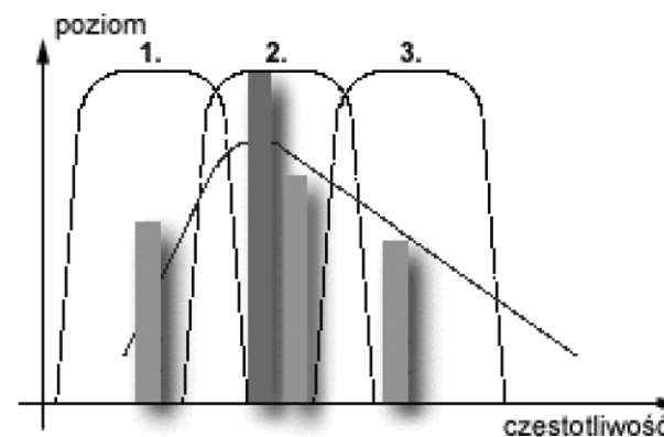
Rysunek 10. Idea działania banku filtrów
