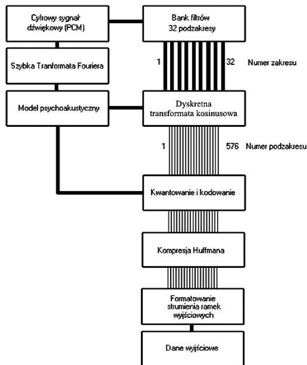
Rysunek 11. Kodowanie MP3
