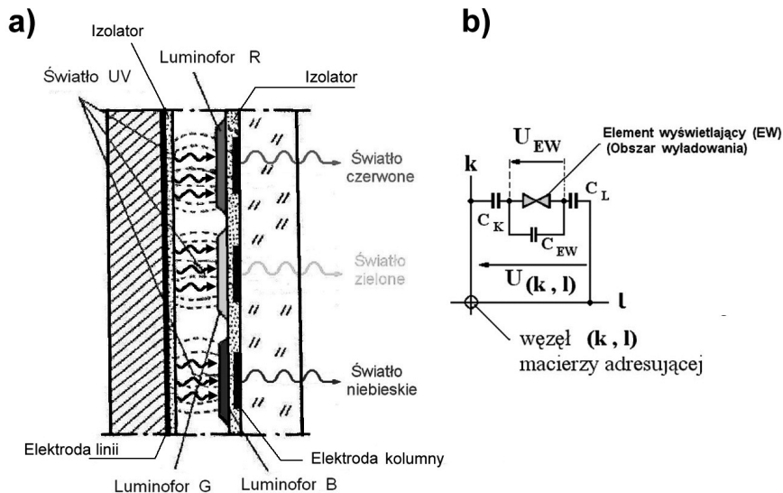
Rysunek 25. Konstrukcja przemiennoprądowego wyświetlacza plazmowego
