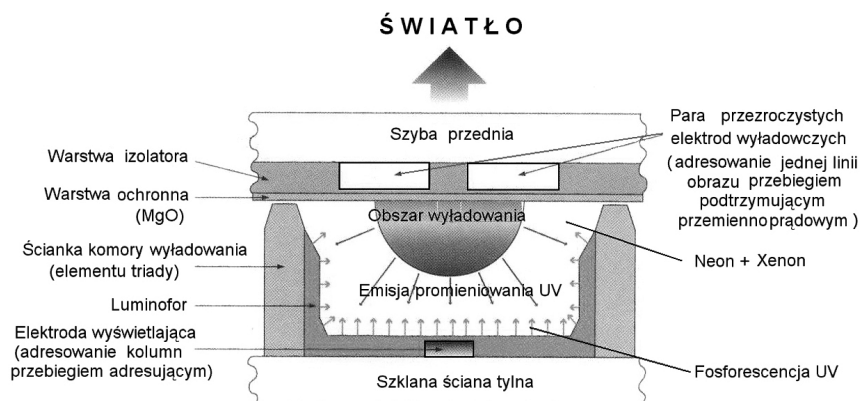
Rysunek 26. Konstrukcja pojedynczego piksela wyświetlacza plazmowego
