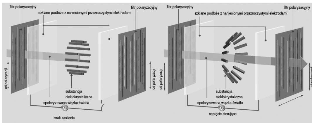
Rysunek 21 Budowa wyświetlaczy LCD wykonanych w technologii MVA
