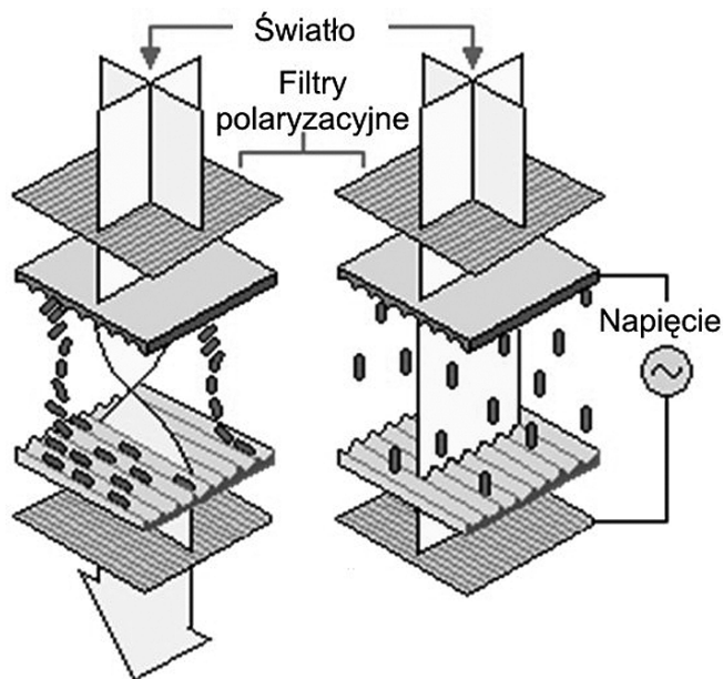
Rysunek 15. Napięcie powoduje zmianę położenia molekuł ciekłego kryształu
