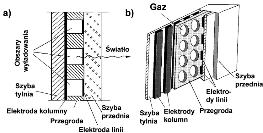
Rysunek 24 Konstrukcja stałoprądowego wyświetlacza plazmowego
