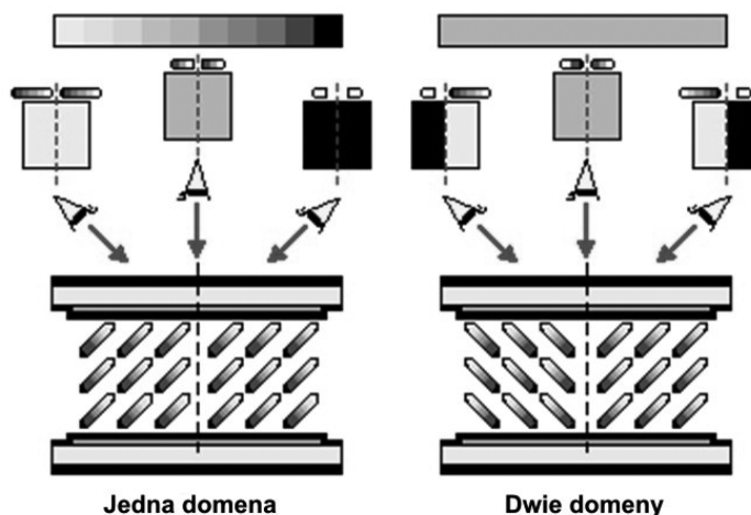
Rysunek 22. Zasada działania matryc MVA
