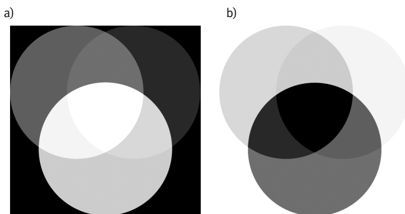
Rysunek 4. Addytywne a) i subtraktywne b) mieszanie barw
