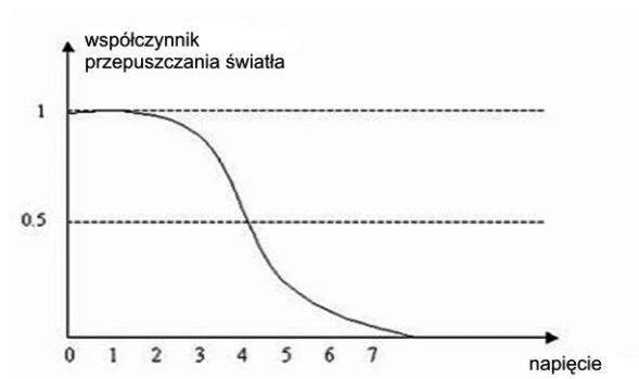
Rysunek 16. Różnicując napięcie na końcówkach ciekłego kryształu można modulować stopień zamknięcia przetwornika, aby uzyskać stany pośrednie
