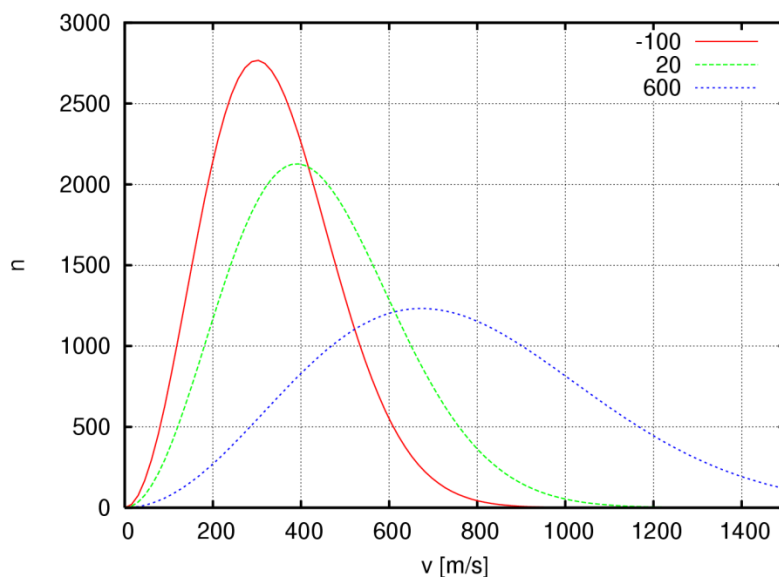
Rysunek 1. Rozkład Maxwella dla tlenu dla trzech temperatur ( -100\text{ }^{\circ}\text{C} , temperatura pokojowa i 600\text{ }^{\circ}\text{C} ). Wartość funkcji odpowiada liczbie cząsteczek spośród 1 miliona cząsteczek, jaka będzie poruszać się z prędkością v \pm 0,5\text{ m/s} (źródło: Wikipedia)
