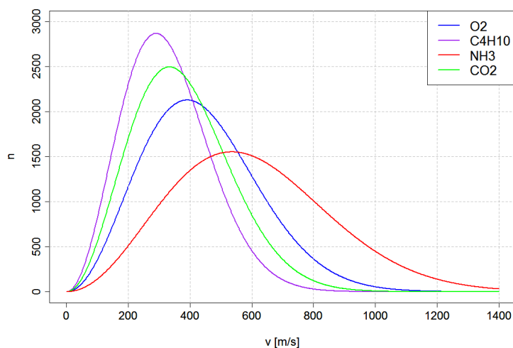
Rysunek 2. Rozkład Maxwella dla tlenu ( O_2 ), butanu ( C_4H_{10} ), amoniaku ( NH_3 ) i dwutlenku węgla ( CO_2 ) w temperaturze pokojowej ( 20\text{ }^{\circ}\text{C} ). Wartość funkcji odpowiada liczbie cząsteczek spośród 1 miliona cząsteczek, jaka będzie poruszać się z prędkością v \pm 0,5\text{ m/s} (źródło: Wikipedia)
