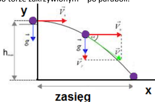
Rysunek 1. Rzut poziomy. Torom ciała jest parabola. Prędkość w kierunku poziomym jest stała przez cały czas. W kierunku pionowym prędkość zmienia się według wzoru v_y = gt
