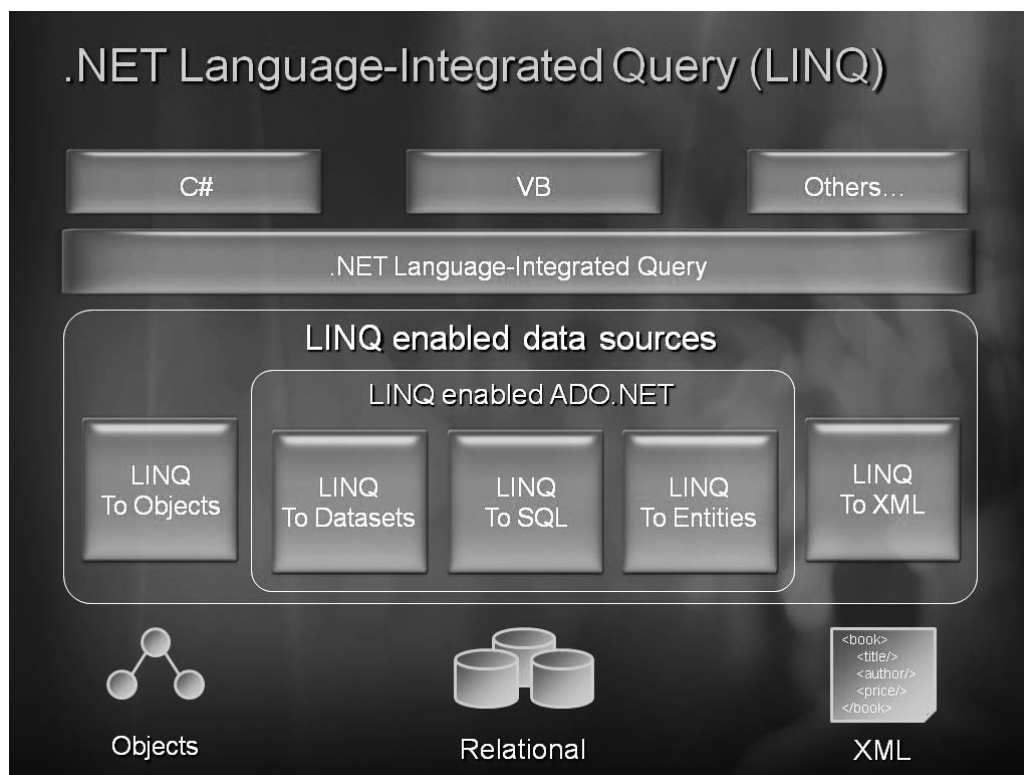
Rysunek 9. Architektura LINQ
